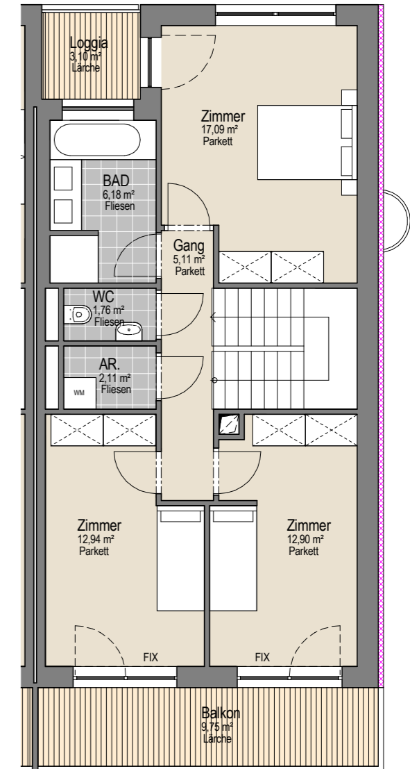
OBERGESCHOSS
